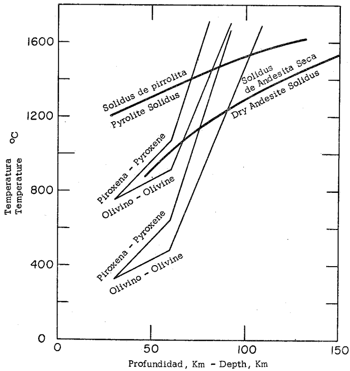
Fig. 3. Geothermas en un manto puro de olivino y de piroxena que corresponde a la zona de baja velocidad de Johnson (1967). Suponiendo temperatura de 330°C y 750°C en la base de la corteza, se deduce fusión parcial por debajo de los 100 Km, aún para un manto seco.
